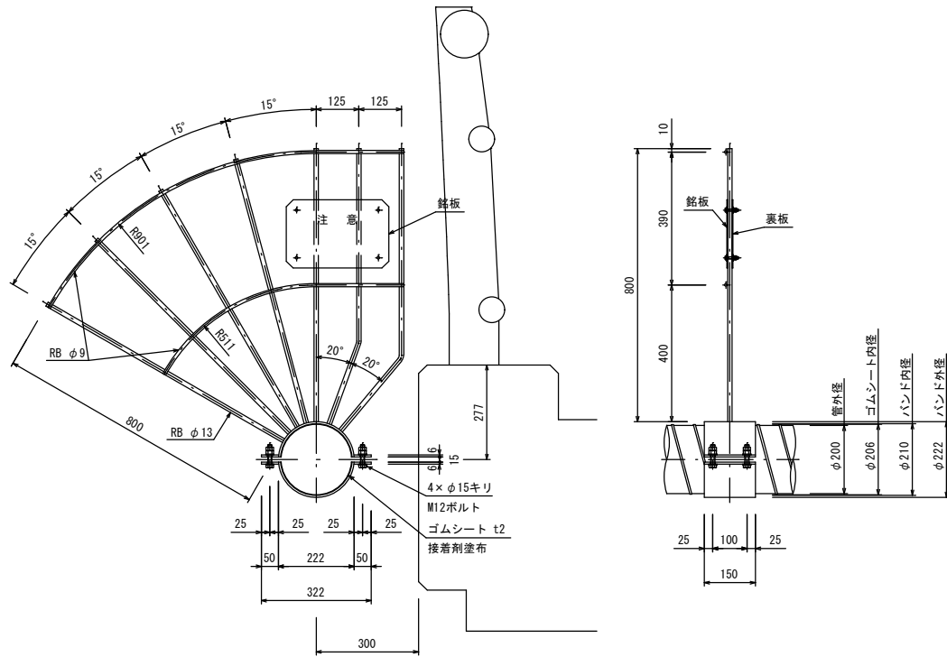
二重管保温工図
