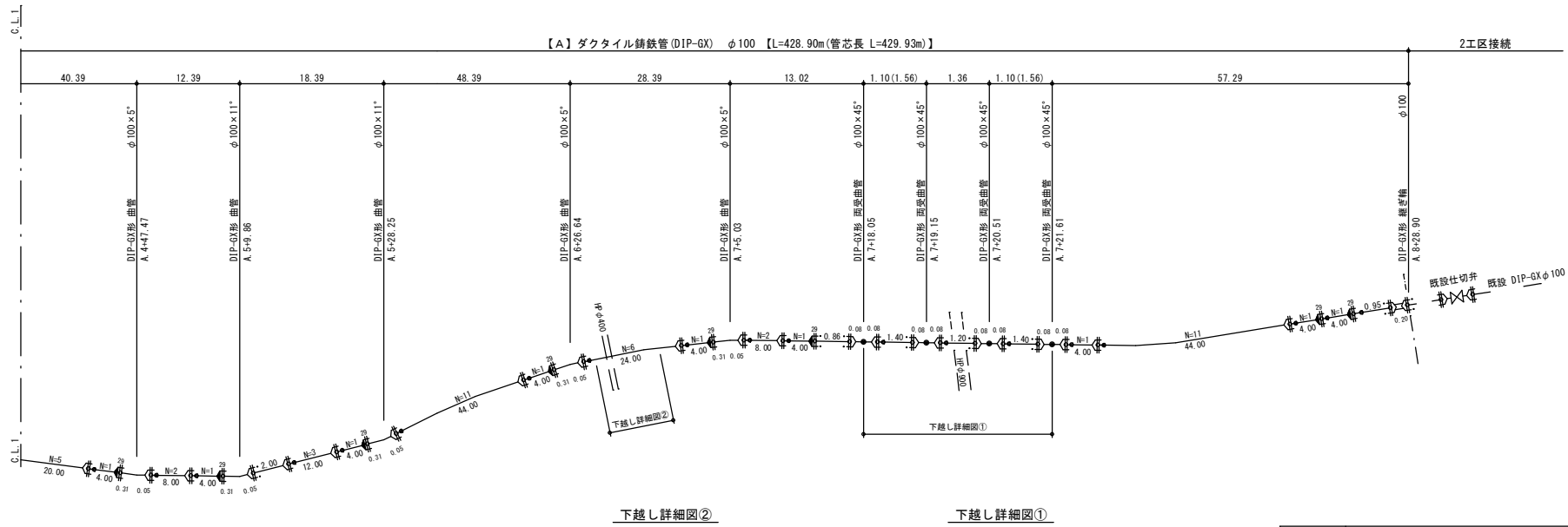
配管詳細図 (2/2)
