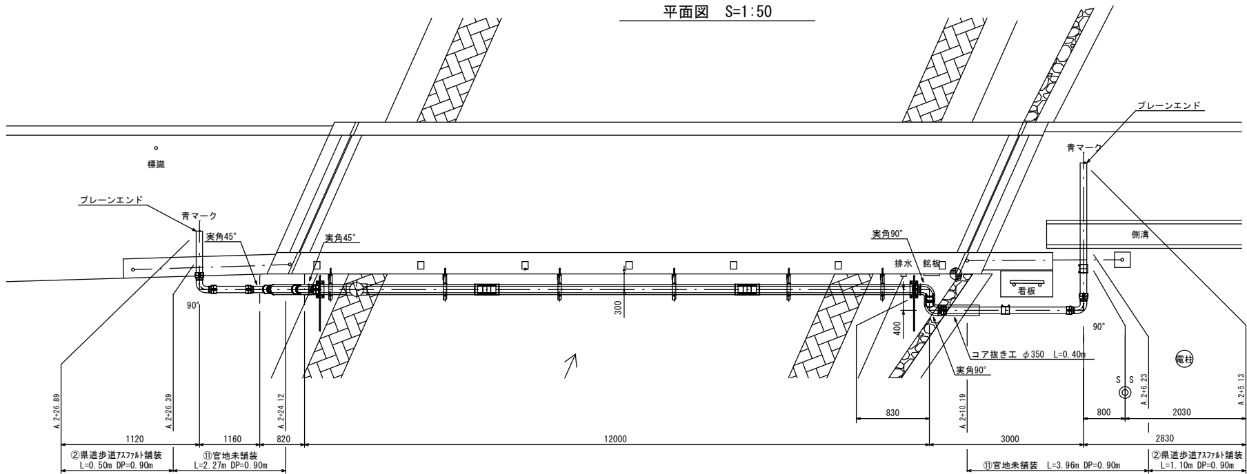
平面図 S=1:50
