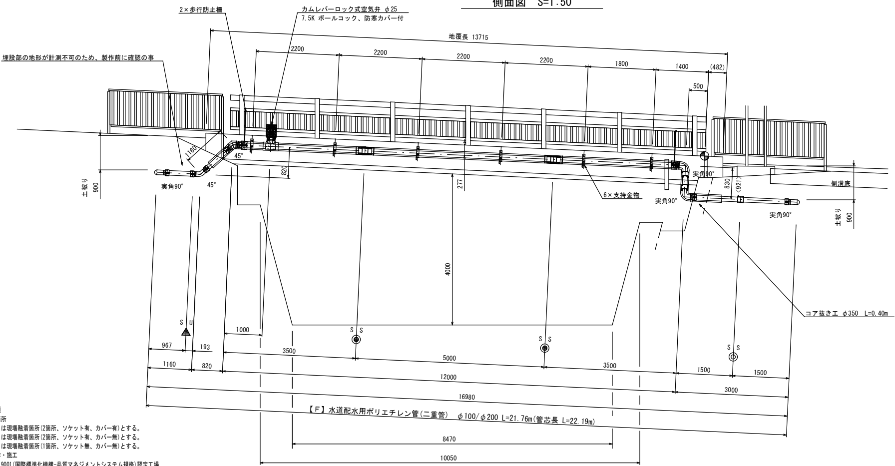
側面図 S=1:50
