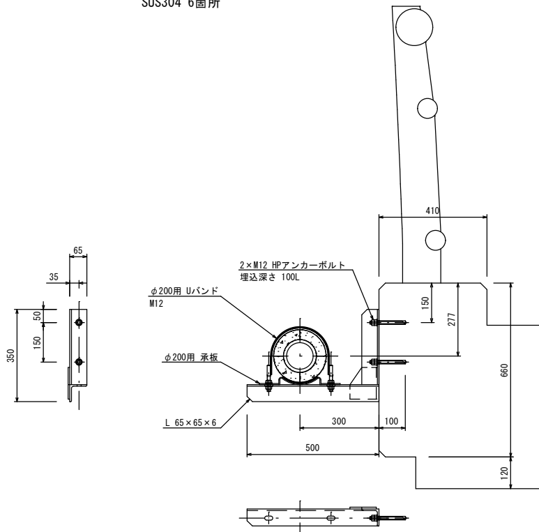
支持金物 S=1:10
