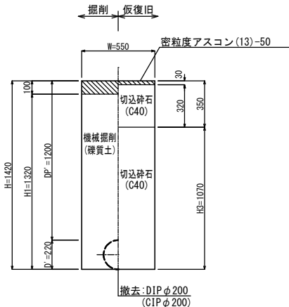
⑤⑧ 県道歩道As (乗入部6.5t以下)
