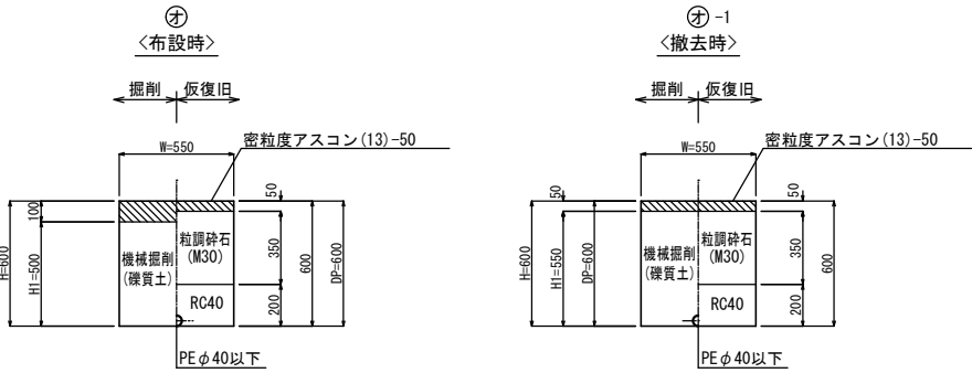
県道車道As
