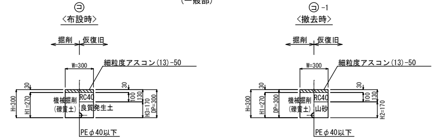
県道歩道As (一般部)
