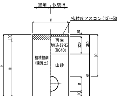
県道歩道As (乗入部6.5t以
