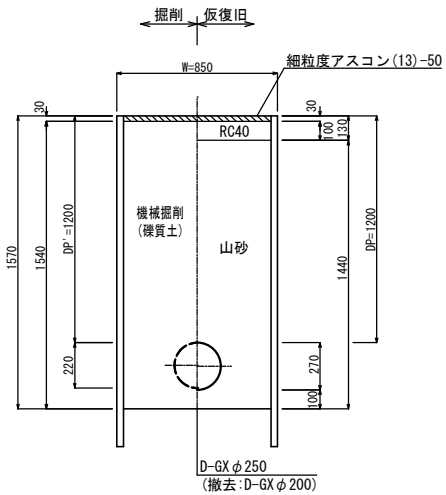
②⑧ 県道歩道As (一般部)
