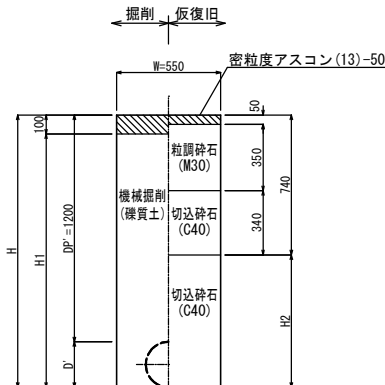
県道車道As
