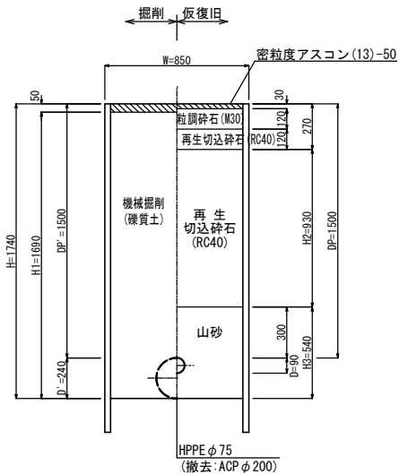
④⑤ 市道車道As 一般市道
