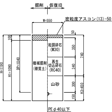
㉑ 県道車道As
