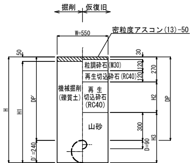
市道車道As 一般市道
