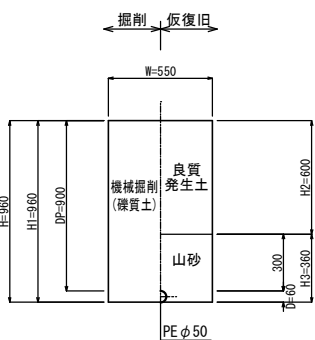
㉜ 宅地内 (砂利)
