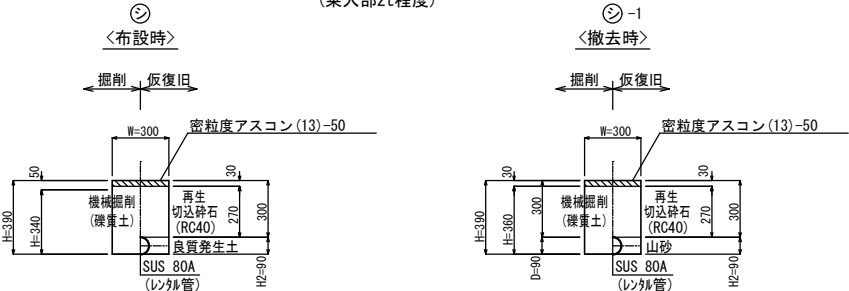
県道歩道As (乗入部2t程度)
