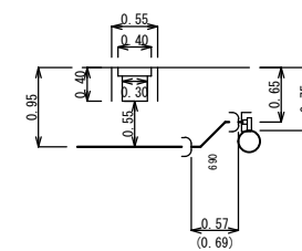
⑥—⑥詳細図 S=1:50
