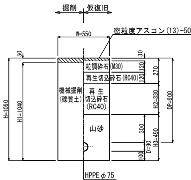
⑪ 市道車道As 一般市道
