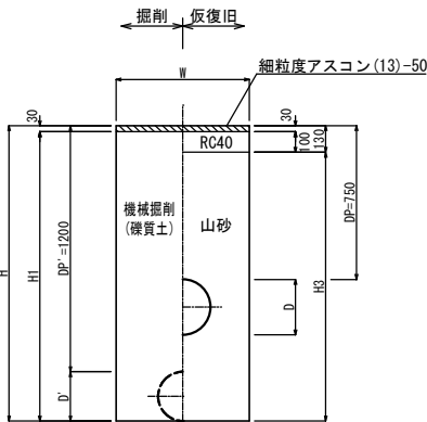
県道歩道As (一般部)
