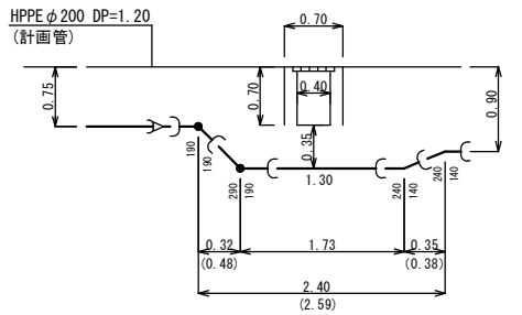
①-①詳細図 S=NON
