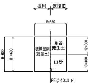
㉞ 宅地内 (ドレン・砂利)
