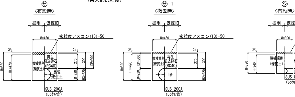
県道歩道As (乗入部2t程度)
