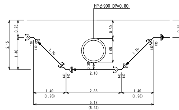
④—④詳細図 S=1:50
