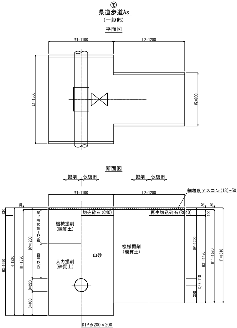
〈不断水 T 字管部〉
