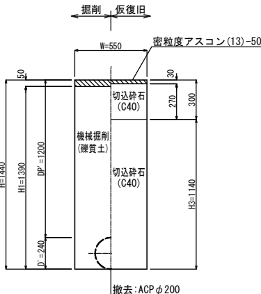
⑤⑦ 県道歩道As (乗入部2t程度)
