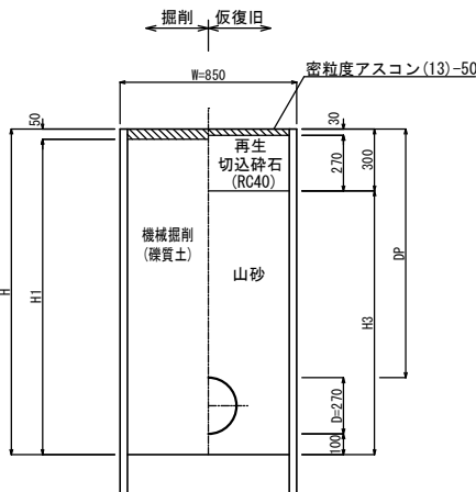
県道歩道As (乗入部2t程度)
