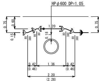
⑬-⑬詳細図 S=1:50
