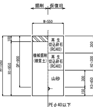
㉘ 市道Co
