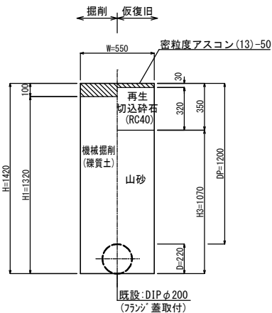
⑮ 県道歩道As (乗入部6.5t以下)
