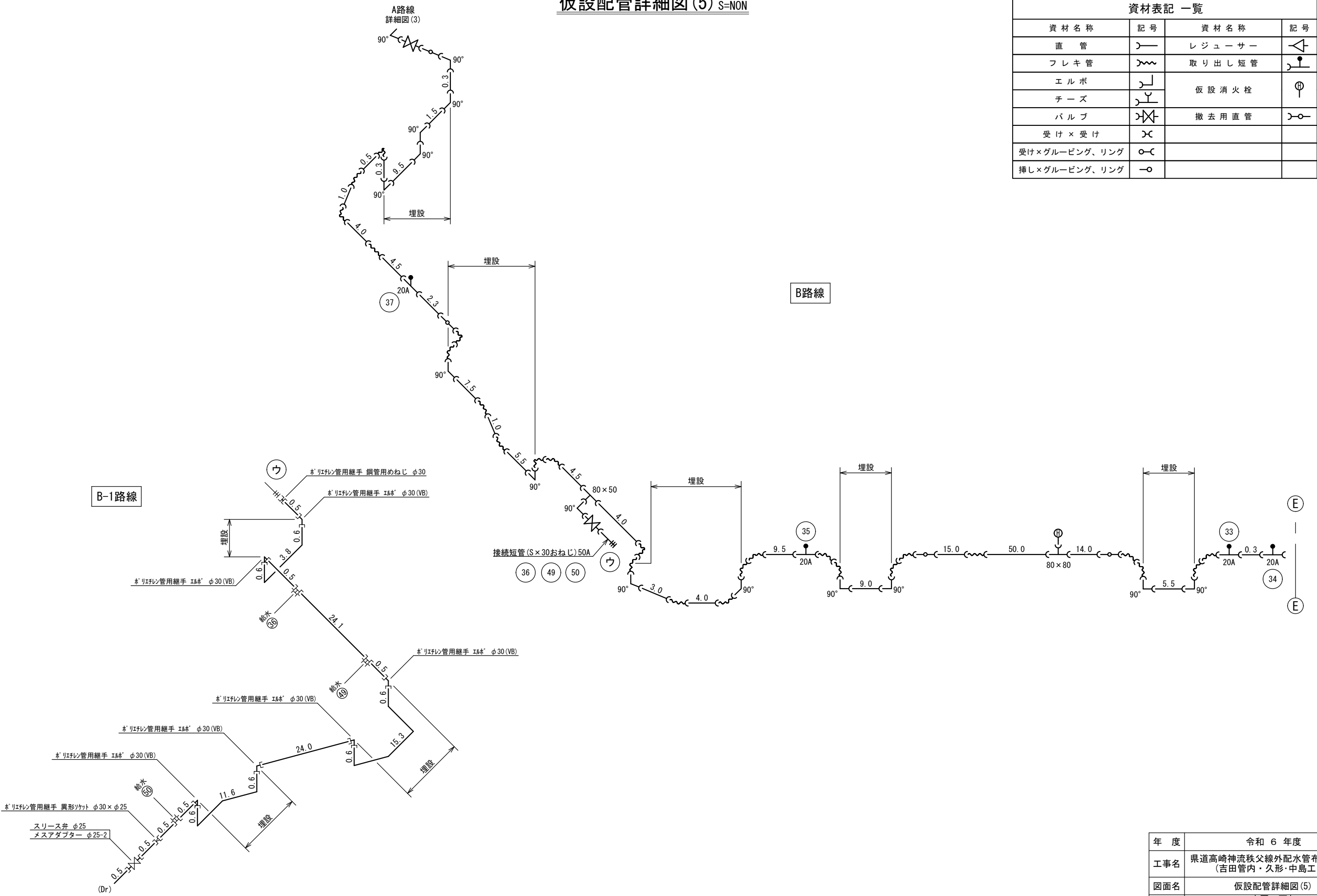
仮設配管詳細図(5) S=NON
