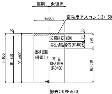
⑥⑩ 市道車道As 一般市道
