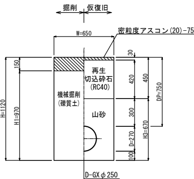
⑬ 県道歩道As (乗入部6.5t超)
