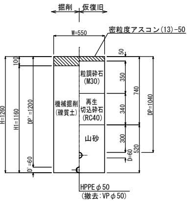
② 県道車道As
