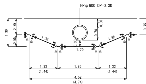
⑤—⑤詳細図 S=1:50
