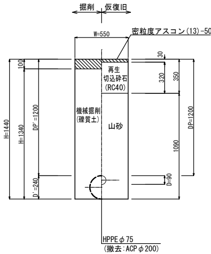
③⑦ 県道歩道As (乗入部6.5t以下)
