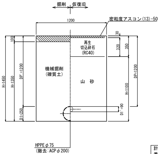
③④ 県道歩道As (乗入部6.5t以下)
