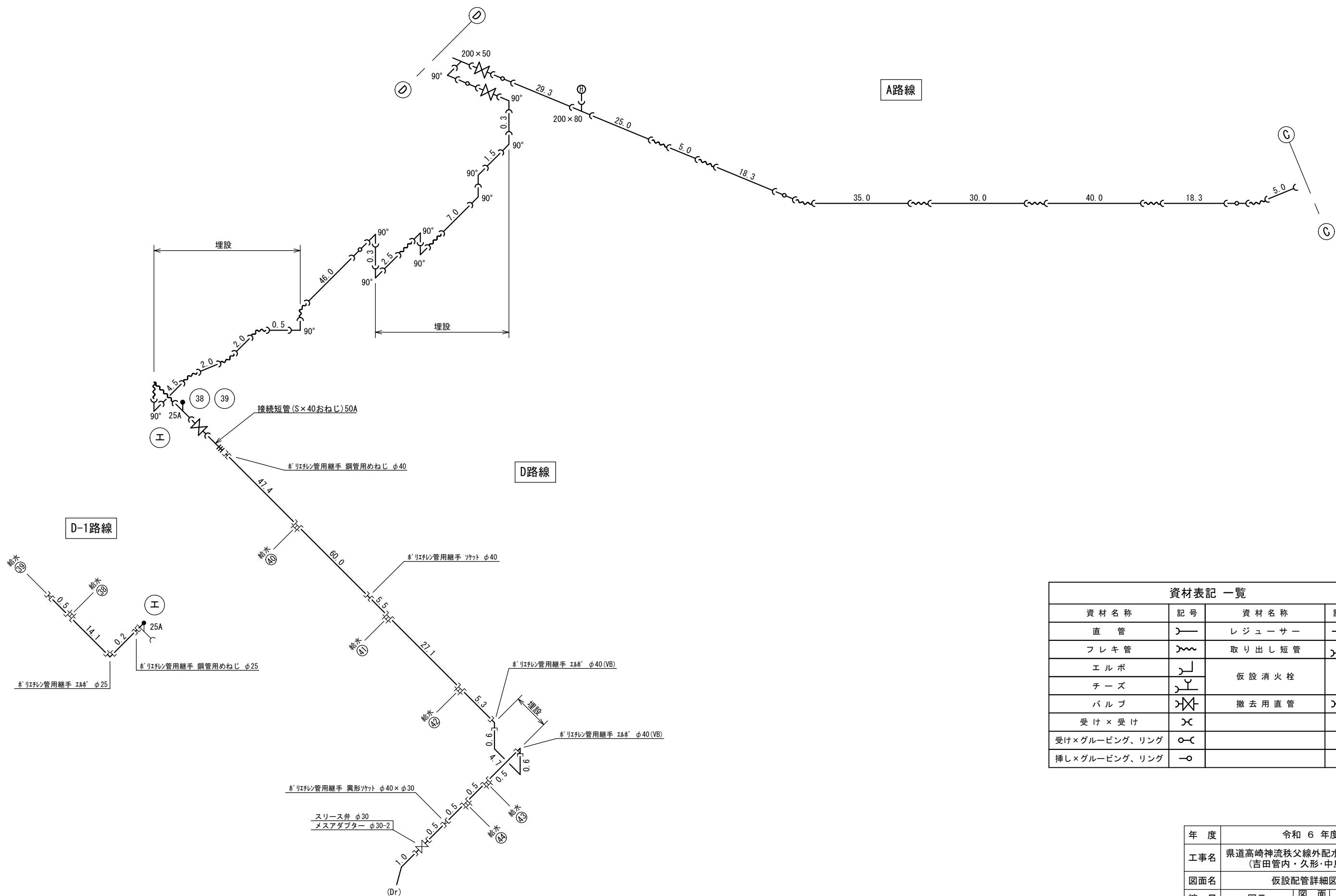
仮設配管詳細図(6) S=NON
