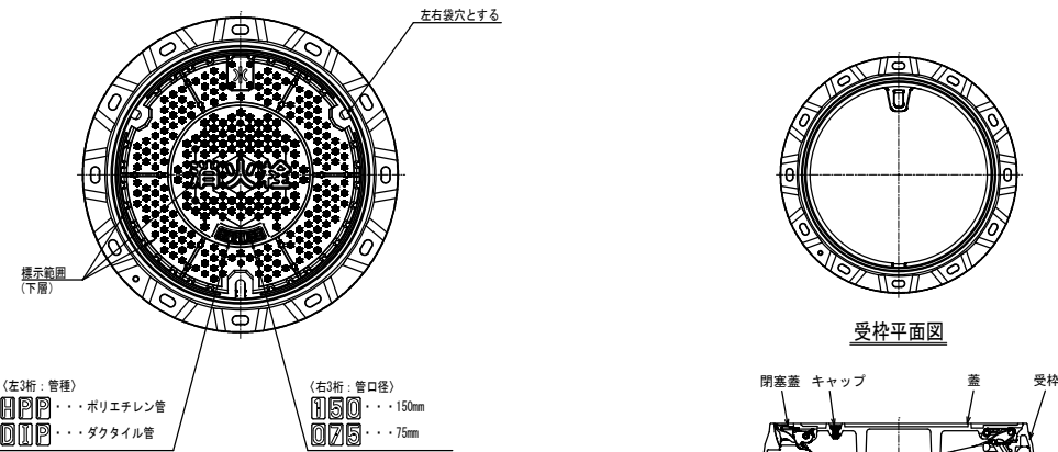
蓋, 受枠平面図
