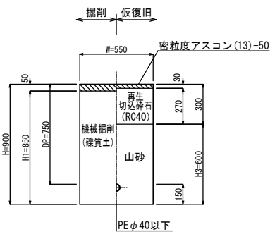
㉔ 県道歩道As (乗入部2t程度)
