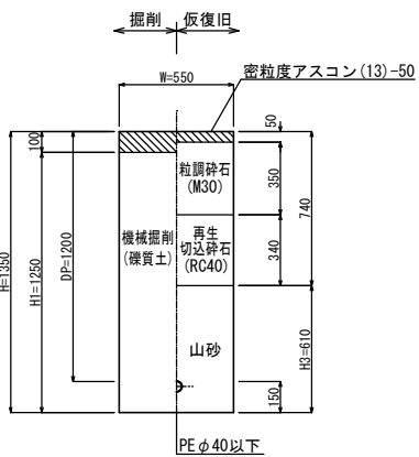
㉒ 県道車道As
