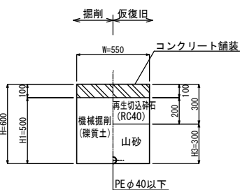
㉛ 宅地内 (Co)
