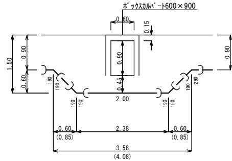
⑪-⑪詳細図 S=1:50
