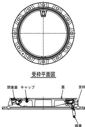
蓋, 受枠断面図
