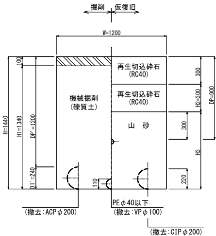
④⑧ 市道Co
