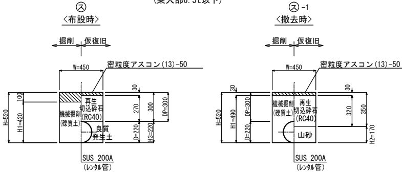
県道歩道As (乗入部6.5t以下)
