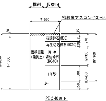
⑮ 市道車道As 一般市道
