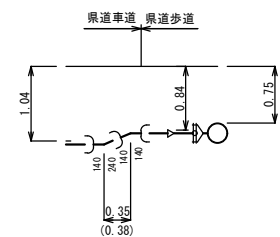
⑫-⑫詳細図 S=1:50
