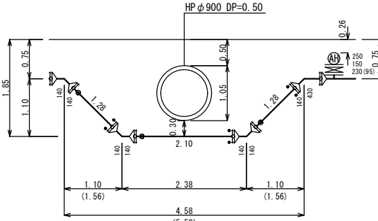
③—③詳細図 S=1:5
