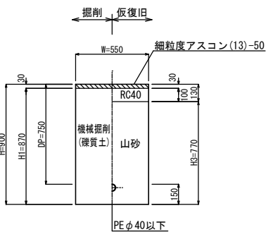
㉓ 県道歩道As (一般部)
