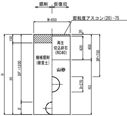
県道歩道As (乗入部6.5t超)
