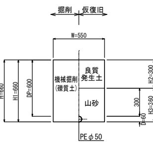
㉝ 宅地内 (砂利)
