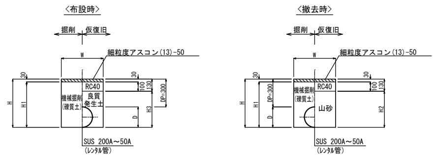
県道歩道As (一般部)
