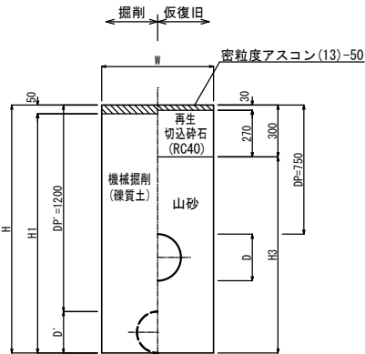
県道歩道As (乗入部2t程度)
