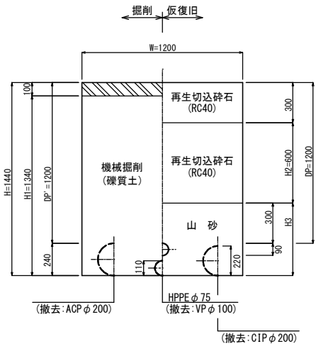
④⑨ 市道Co
