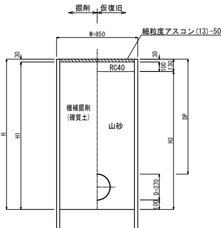
県道歩道A8 (一般部)
