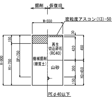
㉖ 県道歩道As (乗入部6.5t超)
