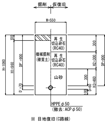
⑤① 市道Co
