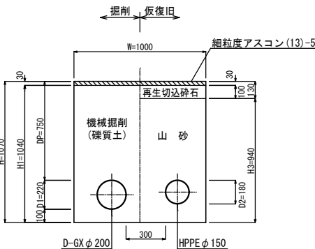
③ 県道歩道As (一般部)
