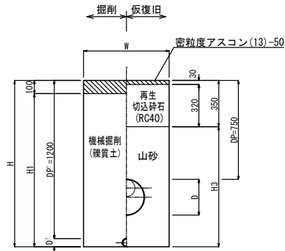
県道歩道As (乗入部6.5t以下)
