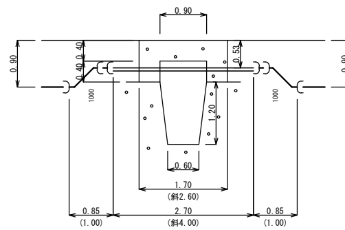
⑦-⑦詳細図 S=1:50
