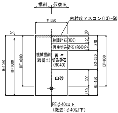
④⑥ 市道車道As 一般市道
