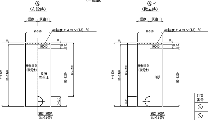
県道歩道As (一般部)
