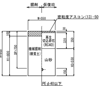
㉕ 県道歩道As (乗入部6.5t以下)
