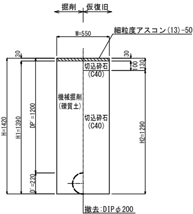
⑤⑥ 県道歩道As (一般部)
